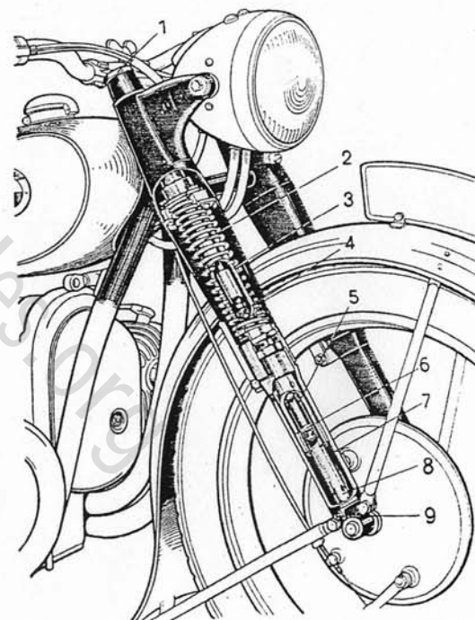
Bild 21. Vorderradgabel
