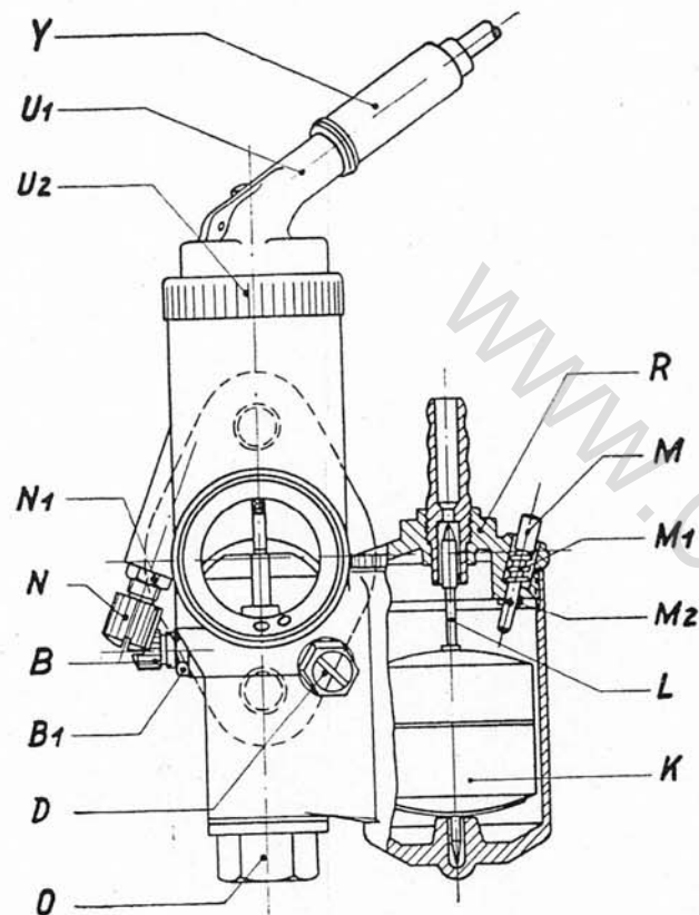
Bild 18. Vergaser R 71
