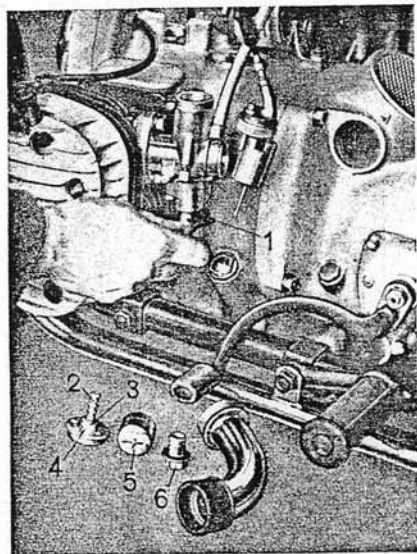
Bild 4. Vergaser R 71
