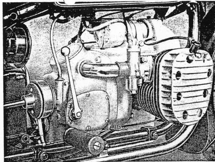
Bild 5. Motoranlage R 71
