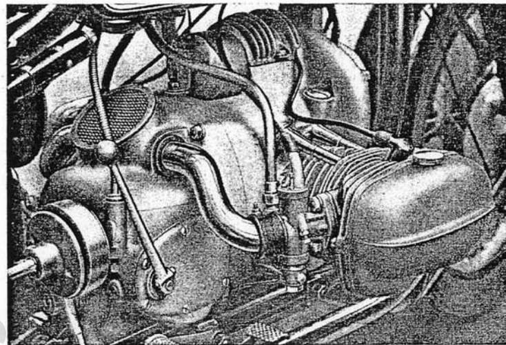
Bild 13. Motorblock R 51
