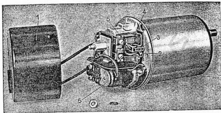
Bild 10. Lichtmaschine
