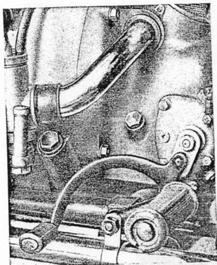
Bild 20. Fußschalthebel
