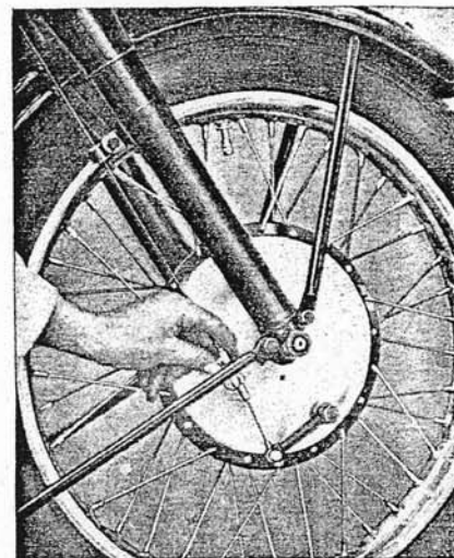
Bild 11. Vorderradbremse
