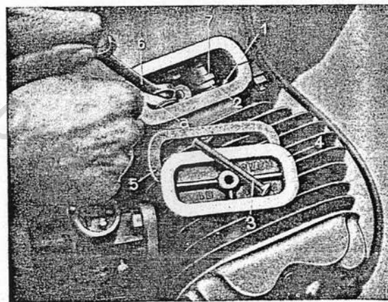
Bild 7. Ventilnachsstellung R 61 (R 71)
