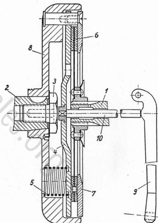
Bild 19. Kupplung
