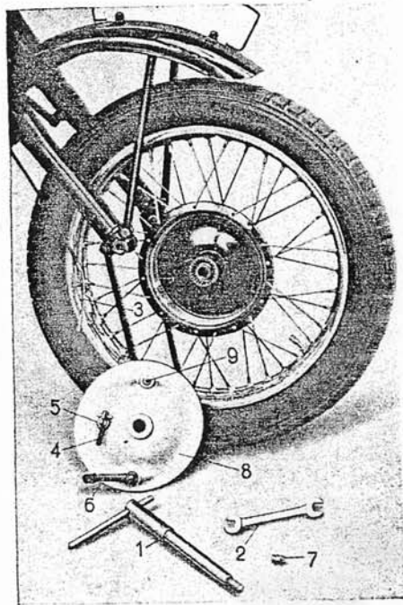
Bild 1. Ausbau des Vorderrades
